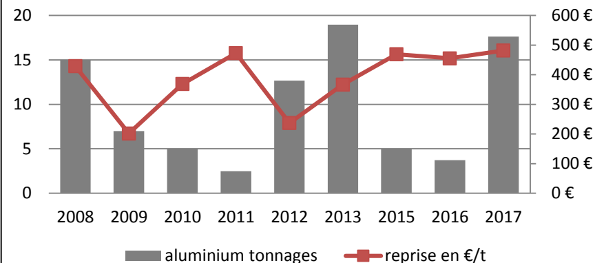
Evolution de l'aluminium (tonnages + prix de reprise)
